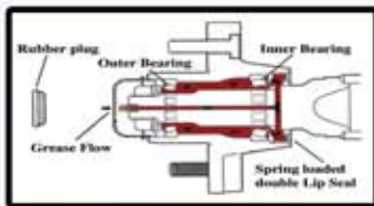
Système de roulements à billes E-ZLUBE (Sur modèles standards) DEXTER AXLE
